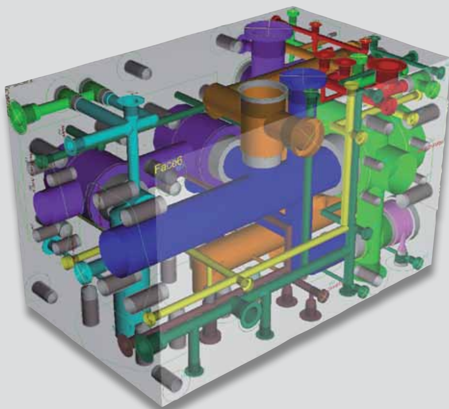
■ طراحی ساختاری یک بلوک کنترل در مرحله برنامه ریزی
